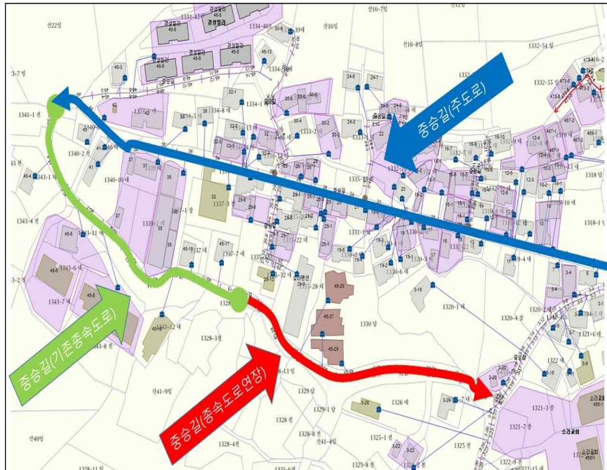
주소정보관리 시스템
